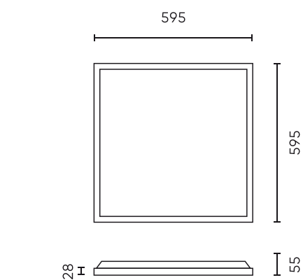
Rysunek techniczny
